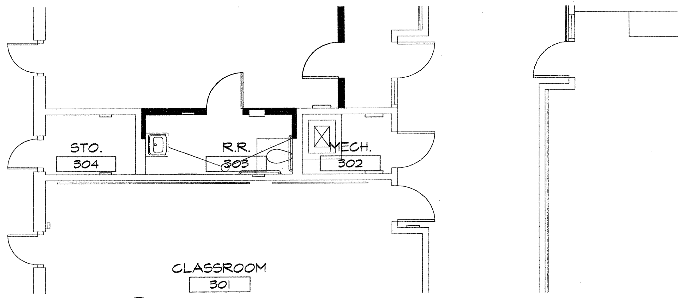
1 ENLARGED FLOOR PLAN SCALE: SCALE: 1/4"=1'-0"
