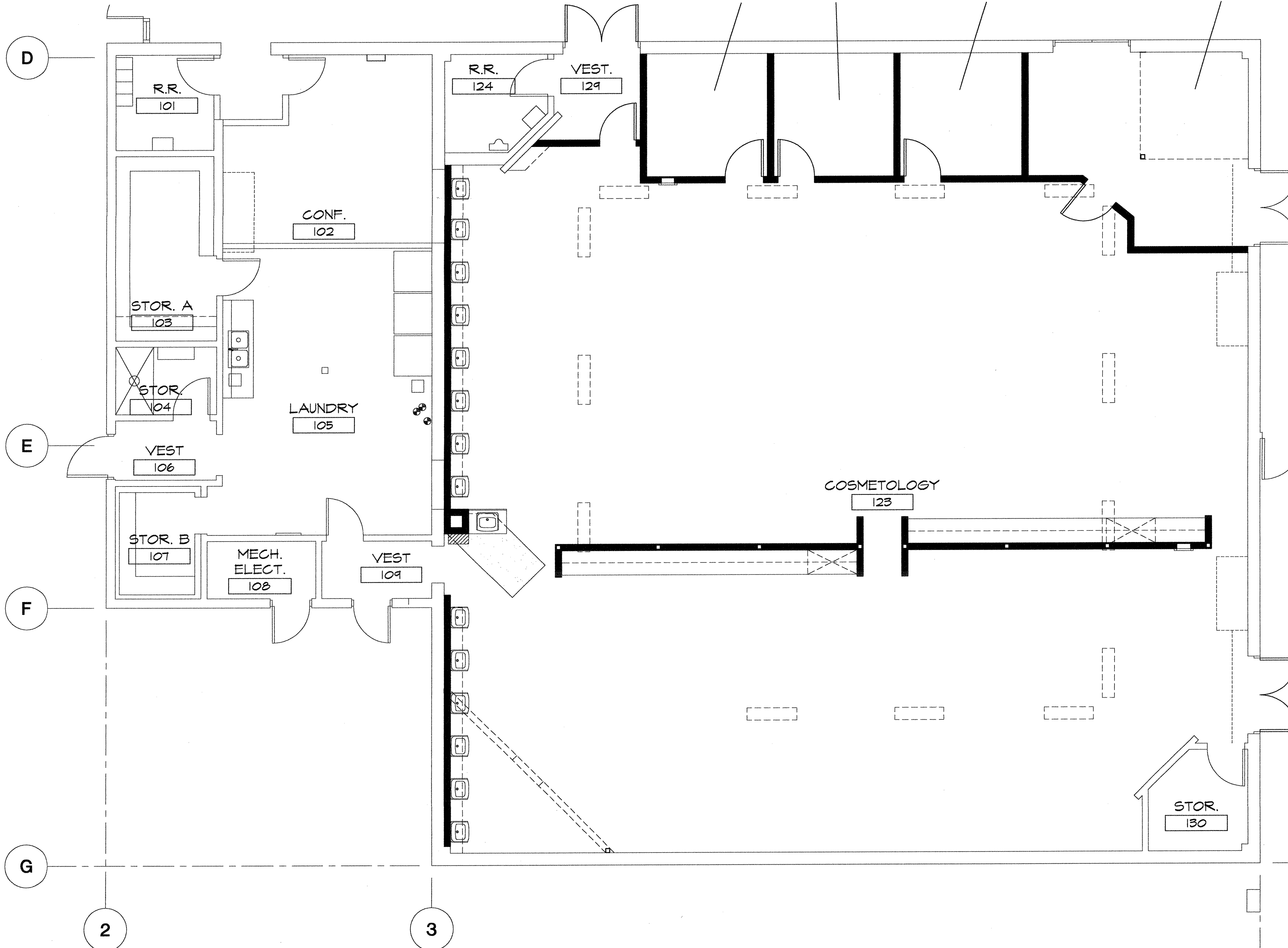
2 ENLARGED FLOOR PLAN SCALE: SCALE: 1/4"=1'-0"
