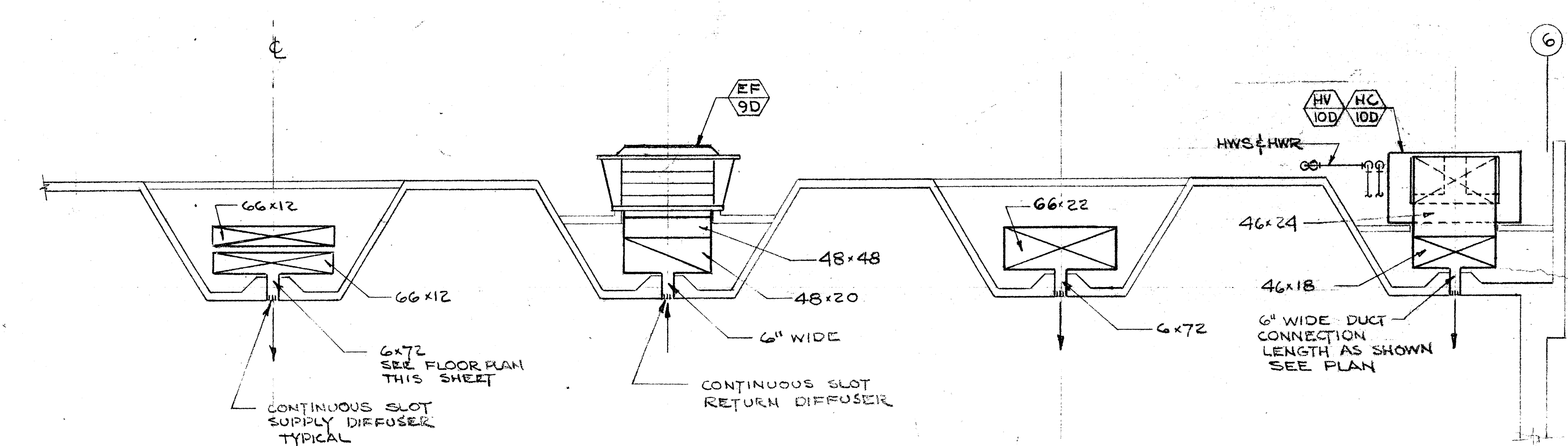
SECTION SCALE: 1/4" = 1'0"
