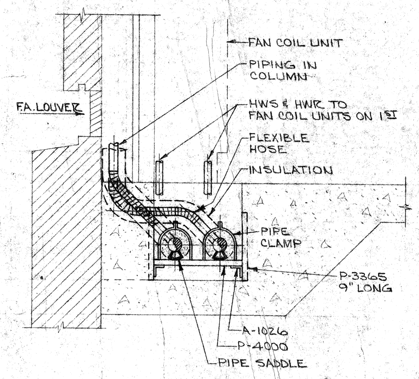
SECTION A-MAA SCALE: 1/2" = 1'-0"
