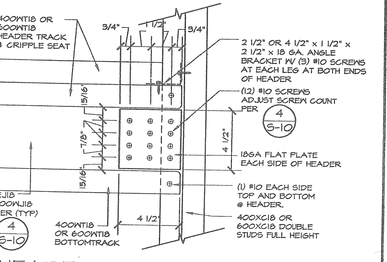
HEADER CONNECTION SCALE: 3" = 1'-0"
